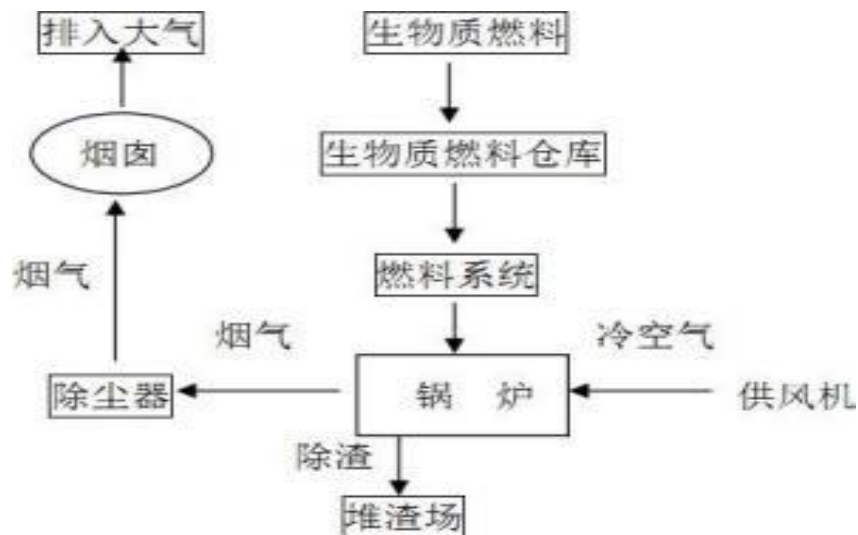
图 2-1 生产工艺流程
